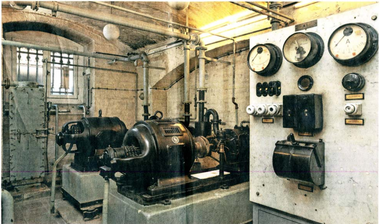
Im Rohrpostkeller des ehemaligen Postamts W 66: Die Anlage im Museum für Kommunikation an der Leipziger Straße war noch bis 1973 in Betrieb.
